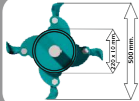
DIAMETRO EJE Ø 60 mm. AXLE DIAMETER Ø 60 mm. DIAMÈTRE DE L'AXE Ø 60 mm. ACHSDURCHMESSER Ø 60 mm.
